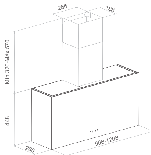
Dimensions en mm Conduits spéciaux sur mesure Conduit d'évacuation des fumées de série sur la version aspirante.
